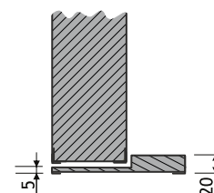
Bundstykke Type 3
